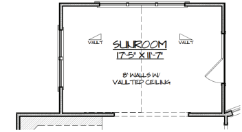
OPTIONAL SUNROOM
