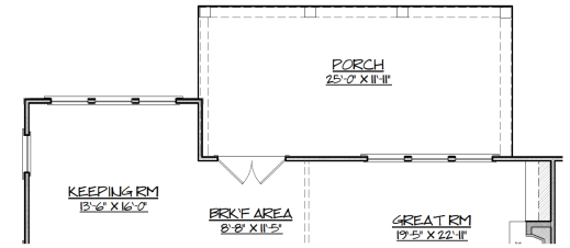
OPTIONAL PORCH
