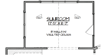
OPTIONAL SUNROOM
